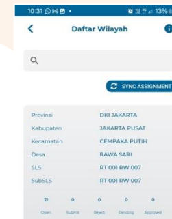
SE2026-P (FASIH)
